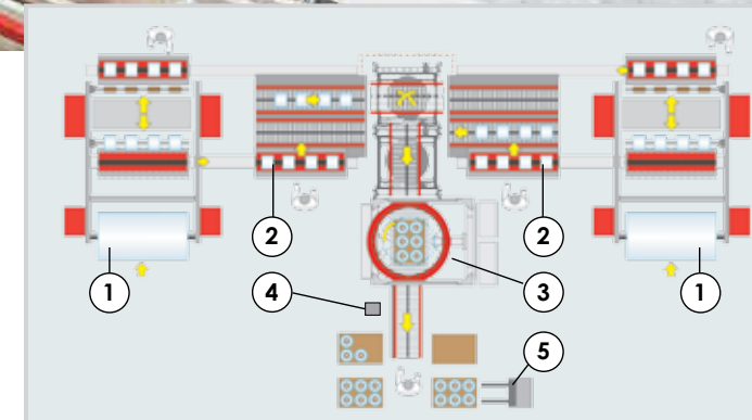
Plant lay-out Lay-out equipo Lay-out fabrika yerleşim planı Anlage lay-out
