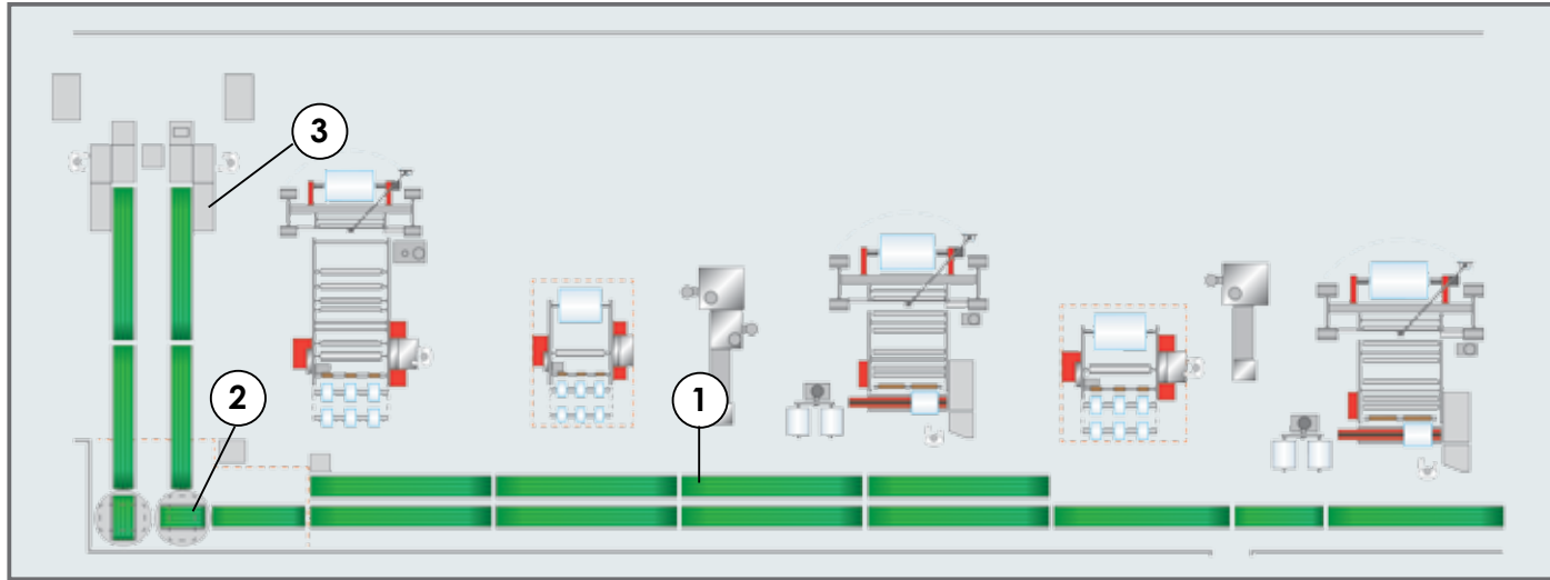
Reel handling & Pallet packing • Transporte bobinas & Unidad de empaquetado • Bobin aktarım ve Paketleme ünitesi • Rollentransport & Verpackungseinheit
